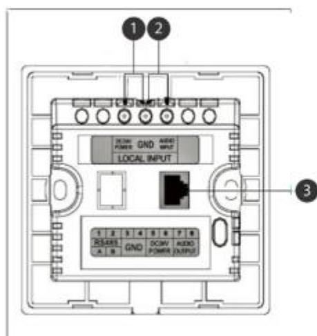
Panel tylny
